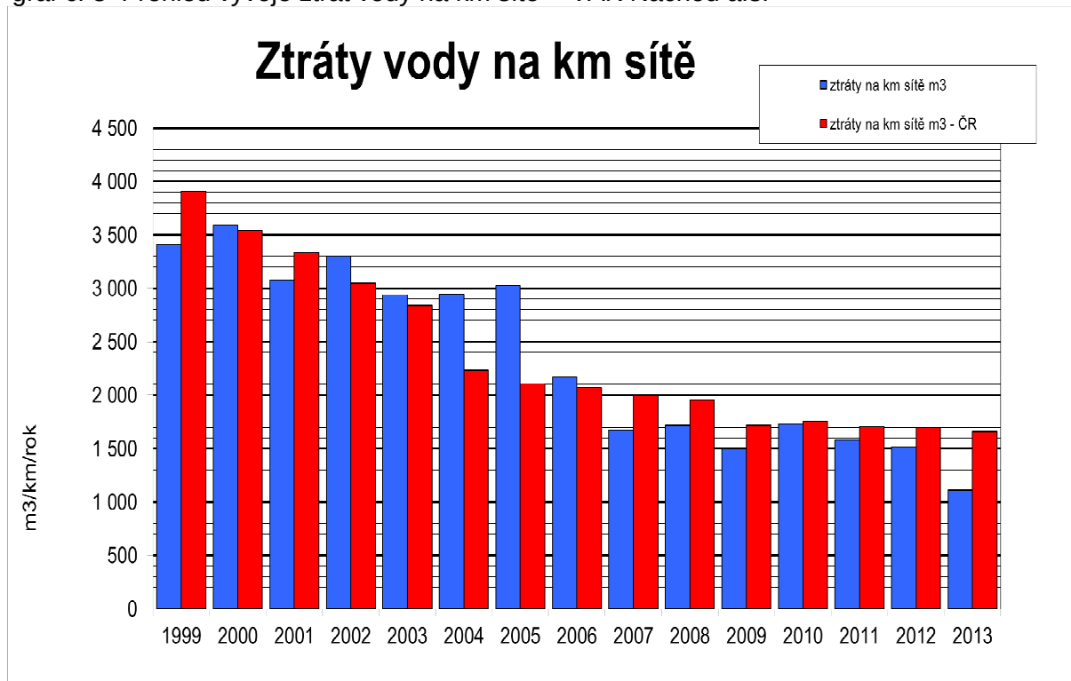
graf č. 8 Přehled vývoje ztrát vody na km sítě - VAK Náchod a.s.
