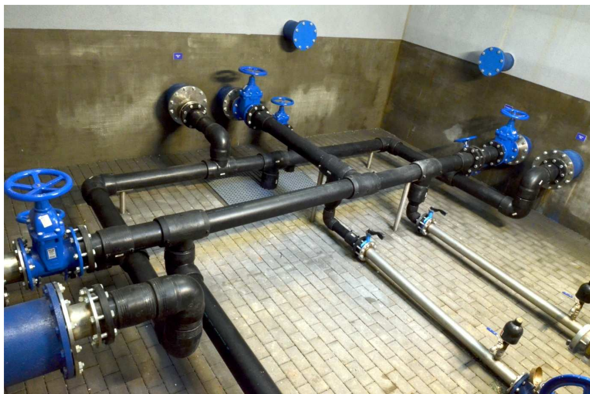
obrázek č.4 Pohled na armaturní komoru VDJ Horka, Bohuslavice nad Metují
